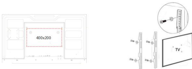
壁挂安装方式示意图
