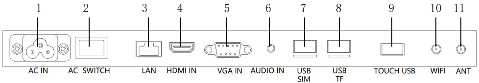
正视图
